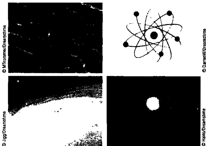
Рисунок 2. Примеры фракталов в природе. Слева — полученное НАСА изображение сверхновой Тихо Браге и изображение вируса риса. Сходство поразительное. Справа — графическое изображение нашей Солнечной системы и изображение модели атома. И те и другие изображения наглядно показывают, как можно использовать себе подобные, повторяющиеся схемы для описания Вселенной — от самой малой ее единицы до самой большой, отличающихся лишь масштабом.
