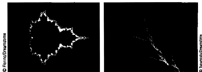
Рисунок 1. В 1970-х годах Бенуа Мандельброт запрограммировал компьютер с целью получить первые фрактальные образы вроде того, который изображен слева. С тех пор ученые установили, что с помощью фрактальной геометрии можно имитировать даже самые сложные схемы природы, такие, например, как лист папоротника (на рисунке справа). Это открытие говорит в пользу той возможности, что природа и Вселенная могут быть результатами или слагаемыми подобных схем, созданных колоссальной квантовой программой, запущенной очень-очень давно.
