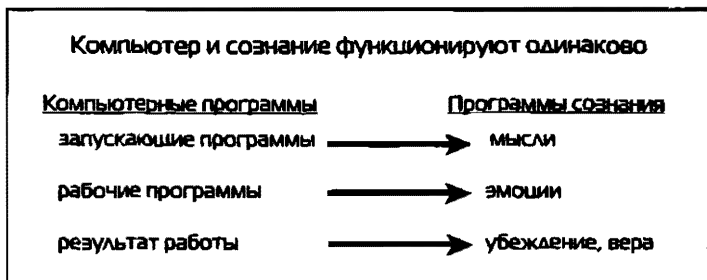
Рисунок 8. Сравнение трех общих элементов в компьютерных программах с их эквивалентами в «программах» сознания Вселенной.
